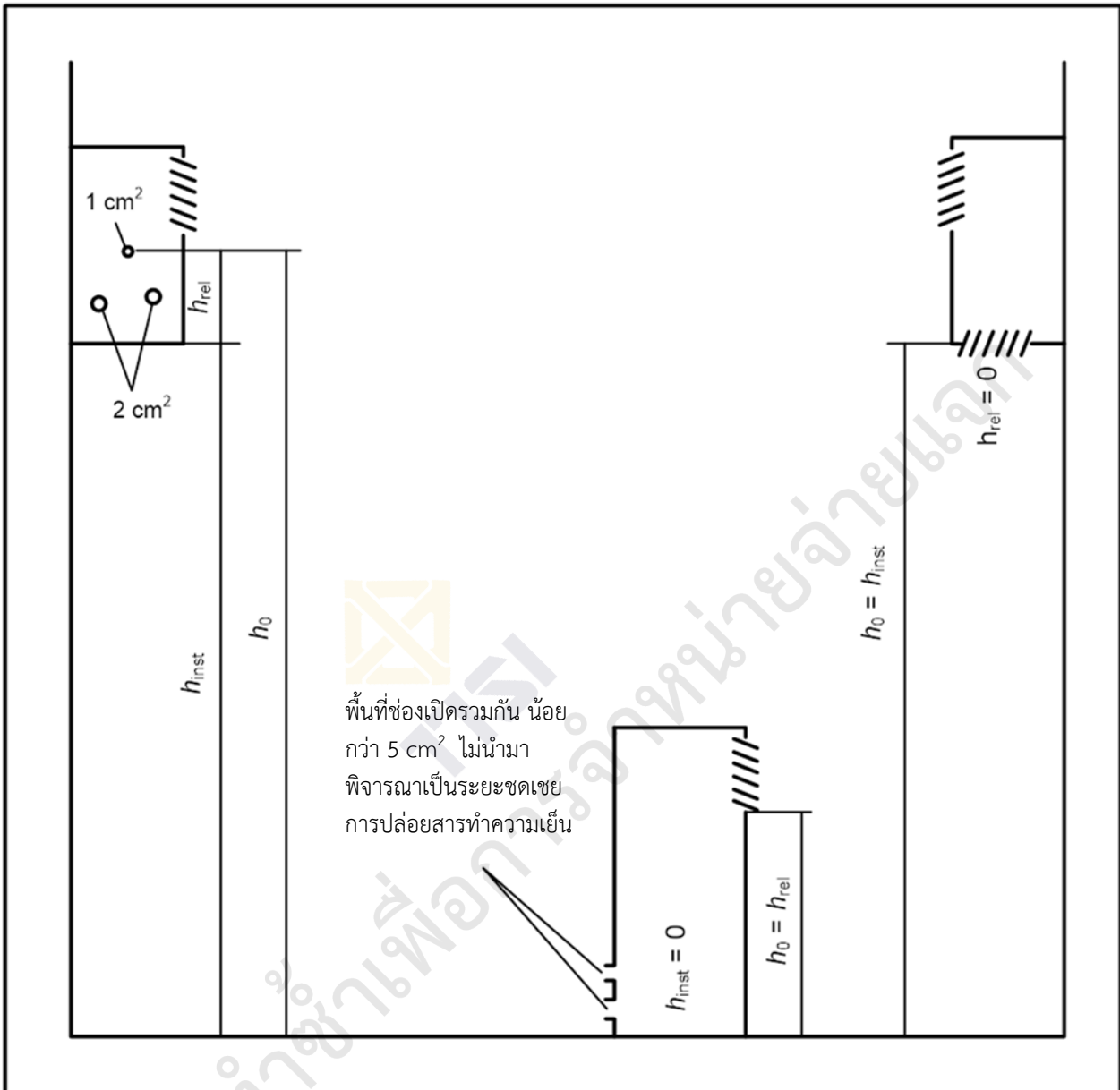
รูปที่ ขข.3 ค่าความสูงของ h_{inst} , h_0 และ h_{rel} สำหรับใช้ในการคำนวณค่า A_{min} และ m_{max}
