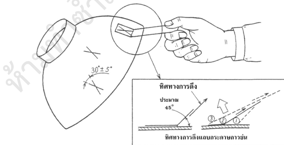
รูปที่ 2 ลักษณะการดึงแถบกระดาษกาวยื่น (ข้อ 8.6.2.3)
