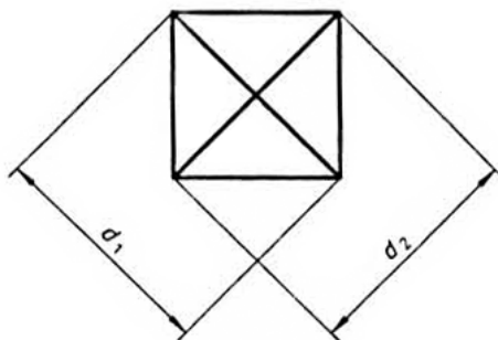
ข) รอยกดวิกเกอร์ส
