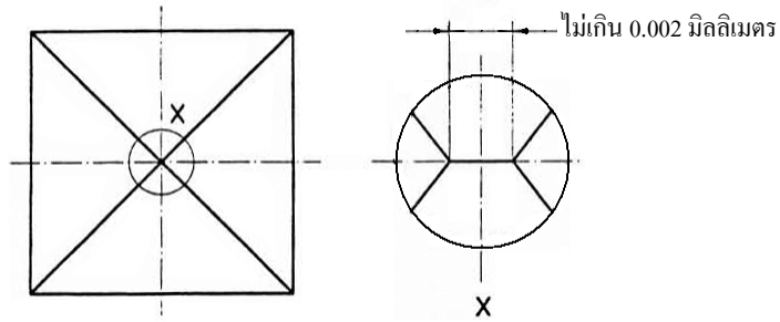
รูปที่ ค.2 เส้นที่ต่อยอดของหน้าเอียง (ข้อ ค.3.2)
